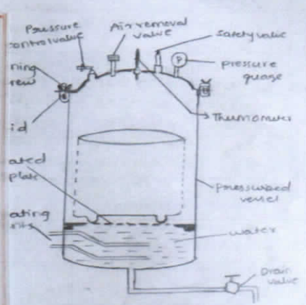
AUTOCLAVE
